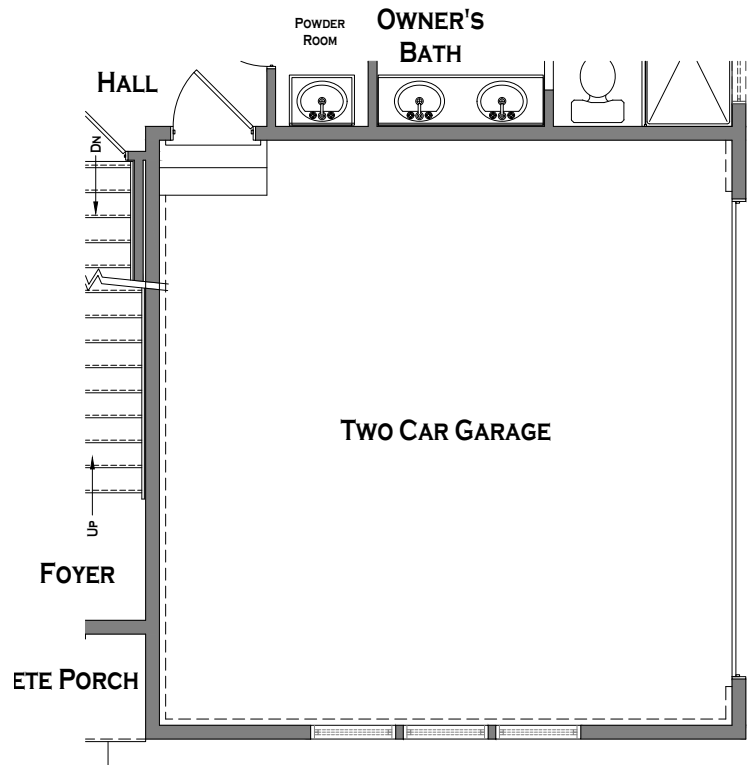
OPTIONAL SIDE LOAD GARAGE
